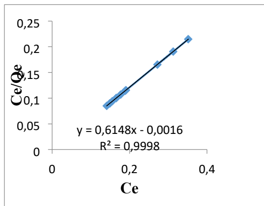
Fig 3 a. Grafik Isoterm Langmuir Freundlich
