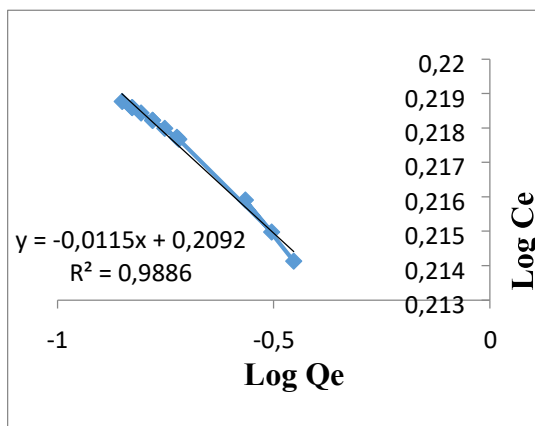
Fig 3 b. Grafik Isoterm
